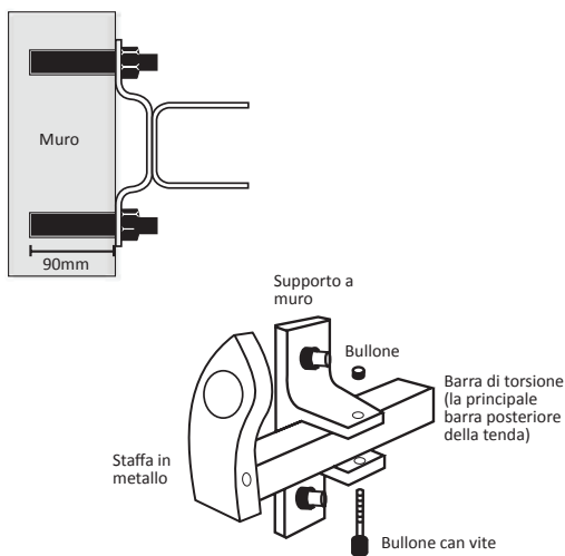
Prospetto laterale - Metodo 1
