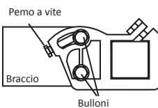
Prospetto laterale - Metodo 1
