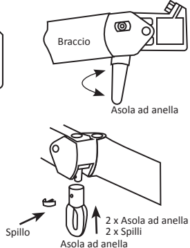
Prospetto laterale - Metodo 2
